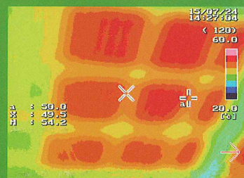
未施工部屋根の裏面温度
